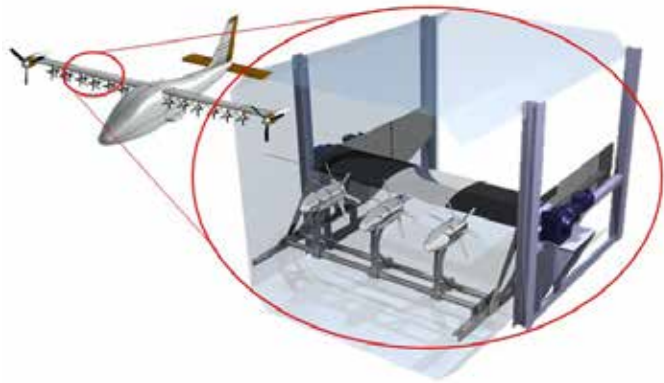
Das Windkanalmodell ist ein Ausschnitt aus einem Flugzeug mit verteilten Antrieben. Bild nach B. Litherland (1)
