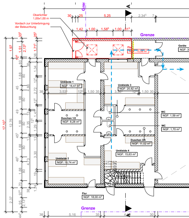
Ausschnitt aus dem Bauantrag (Zeichnung wird gerade noch einmal überarbeitet). Eingezeichnet ist zudem die neue Haupteinschließung für die Hallennutzung.
